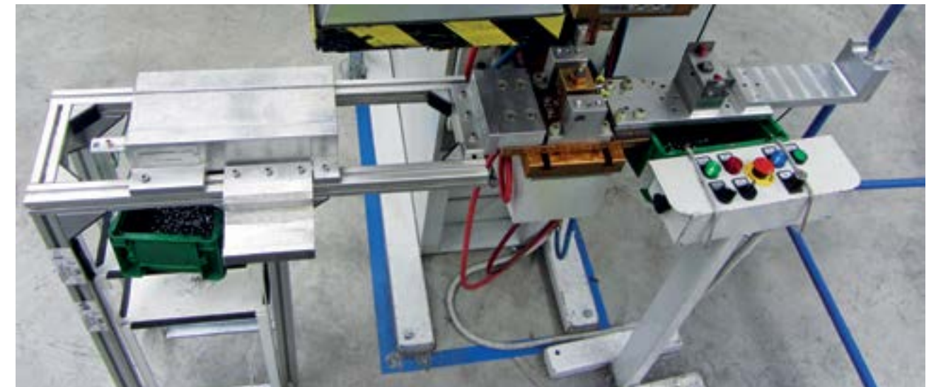
Gutes Beispiel für eine Prozessverbesserung: Durch eine einfache, aber sehr effiziente Modifikation an den Montagegestellen einer manuellen Presse konnte die Rüstzeit von 20 auf 3 Min. verkürzt werden.
