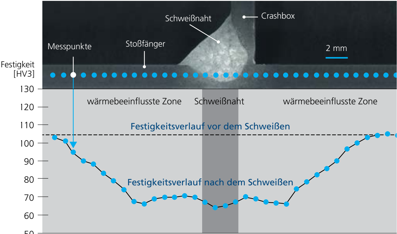
Abb. 3: Typischer Festigkeitsverlauf im Bereich der wärmebeeinflussten Zone einer Schweißnaht für eine hochfeste Aluminium-Crashlegierung
